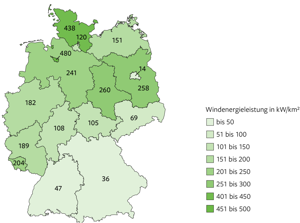
Installierte Windenergieleistung in den Ländern pro Fläche in kW/km 2 (Stand: 30.06.2021)
