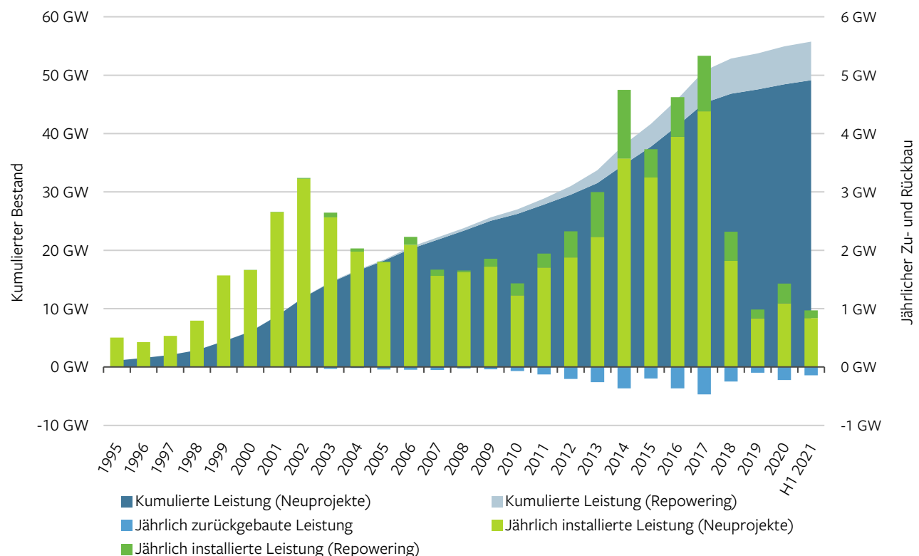
Windenergieleistung an Land in Deutschland und deren jährliche Änderung (Stand: 30.06.2021)
